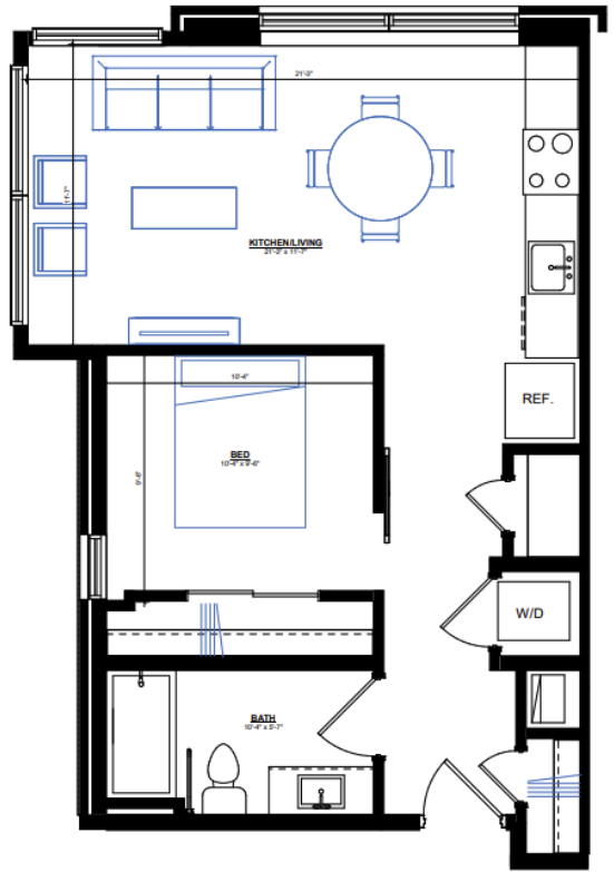
1 SUITE 111 SCALE: 1/2" = 1'-0"
