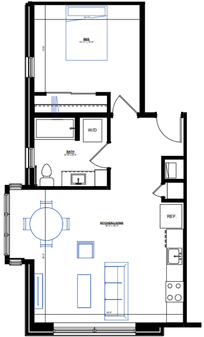
1 SUITE x12 SCALE: 1/2" = 1'-0"
