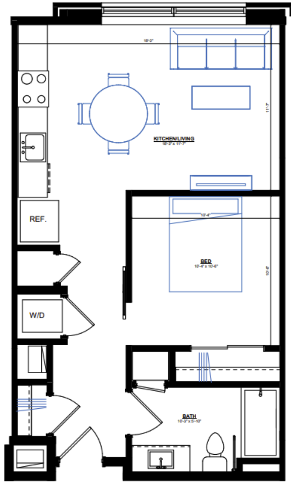
1 SUITE x05, 206, 306, 406, x07, x08, x09 SCALE: 1/2" = 1'-0"
